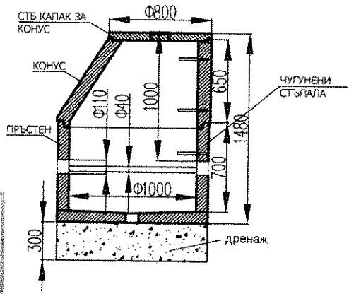
РЕВИЗИОННА ШАХТА С КОНУС И СТЬ КАПАК (извън населено място)
