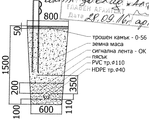
Детайл на при пресичане на път
